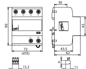
rysunek wymiarowy DVA CSP 3P 100 S FM
